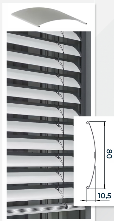
C 80 GEBÖRDELTE LAMELLE
