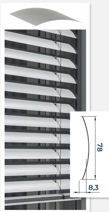
F 80 FLACHLAMELLE
