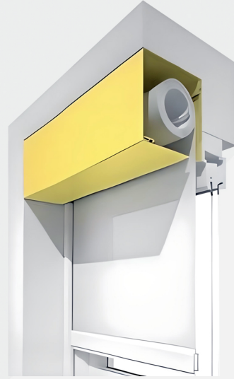
ZipTex KASTEN 90° (Revision vorne/unten)
